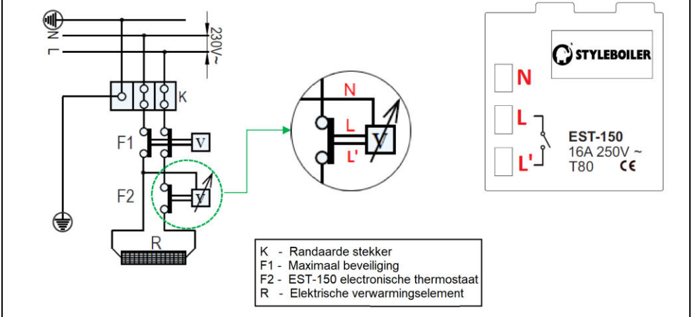
Afbeelding 28 – Elektrisch bedradingschema
